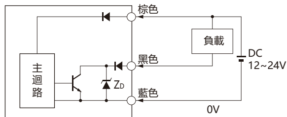
NPN
