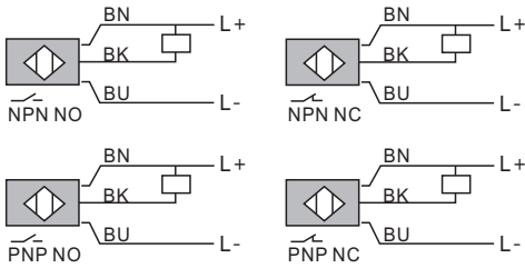
芯綫顏色 BN棕色 BU藍色 BK黑色
