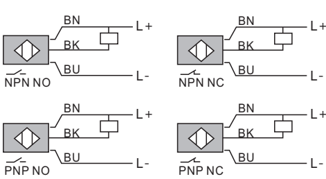
芯線顏色 BN棕色 BU藍色 BK黑色
